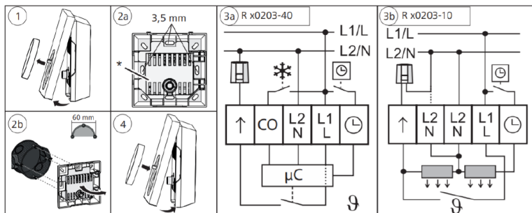
Huonetermostaatin kytkentä suoritetaan kuvan 3a tai 3b mukaisesti.
